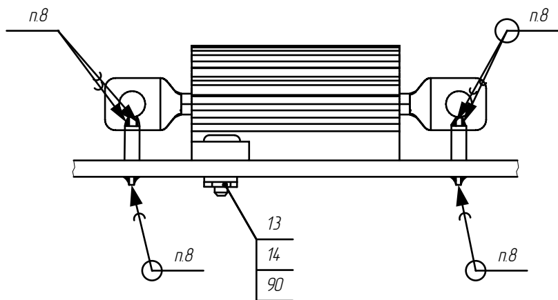
Установка R68, R69
