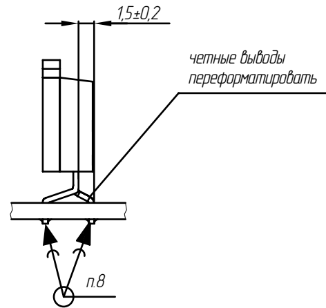
Установка DA15, DA16
