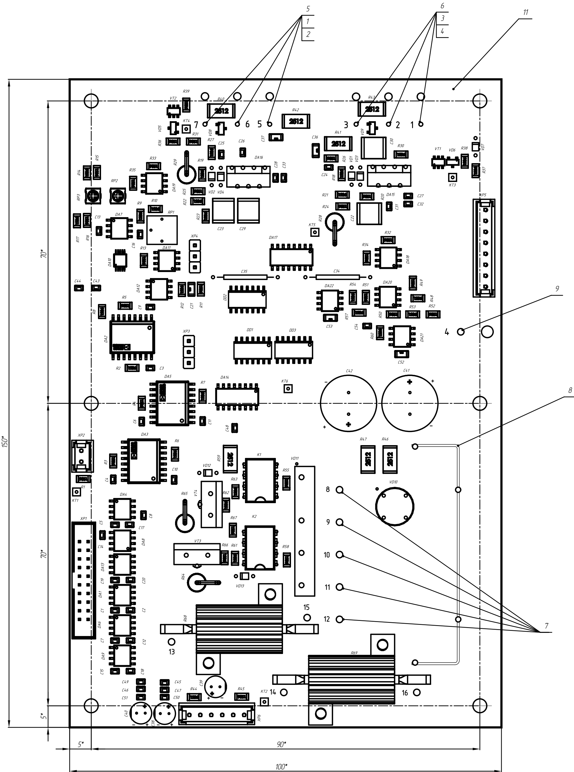
Установка DA15, DA16
